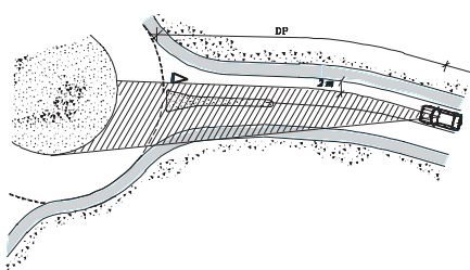
Figura 23 - Critério mínimo de visibilidade na aproximação
