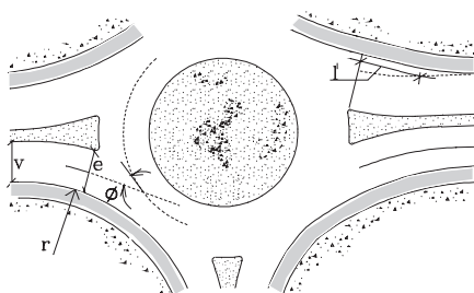
Figura 11 - Parâmetros geométricos da entrada
