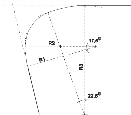
Figura 15 - Curvas compostas
