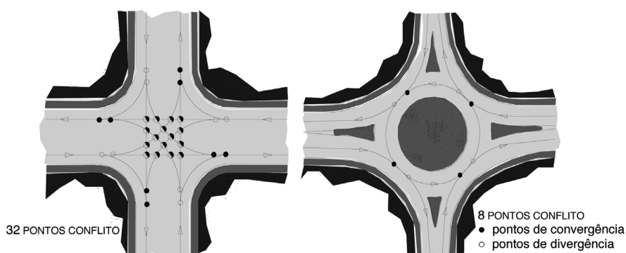
Figura 1 - Pontos de conflito em Cruzamentos Prioritários /Rotundas
