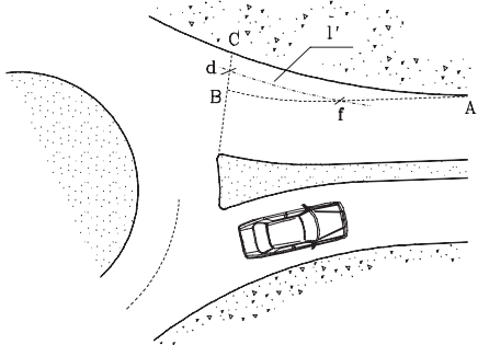
Figura 13 - Medição do comprimento efectivo do leque (l')
