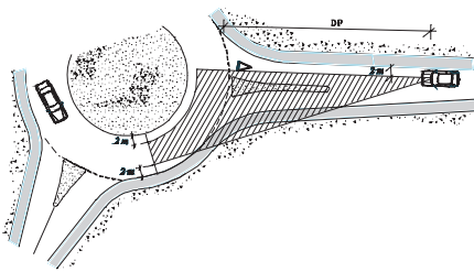
Figura 22 - Critério de visibilidade de aproximação (recomendável para situações ideais de circulação)
