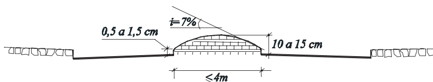
Figura 21 - Perfil transversal de uma Mini-rotunda - pormenor da ilha central
