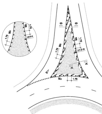
Figura 43 - Ilhéu separador, guias e marcadores (fonte Almeida Roque, 2004)
