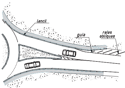
Figura 35 - Definição de passeios em zona urbana, com supressão de bermas
