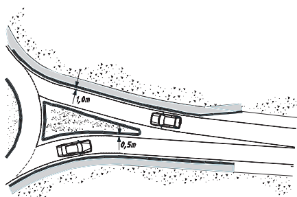
Figura 33 - Definição de passeios em entradas com ilhéu separador
