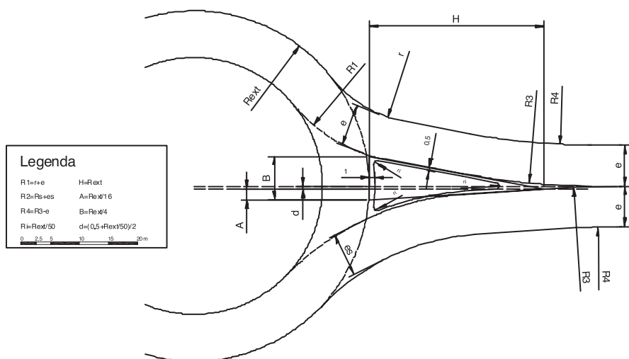
Figura 18 - Traçado do ilhéu separador - Rotundas com raio exterior superior a 15 metros (SETRA, 1998)
