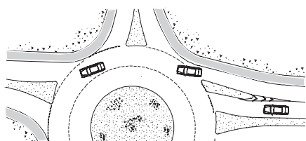
Figura 29 - Uso de ilhéus deflectores complementares
