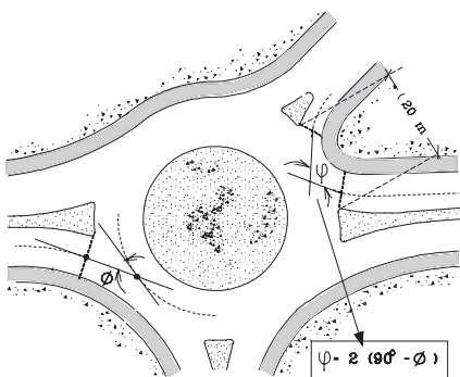
Figura 14 - Processo de medição do ângulo de entrada ( \varphi )
