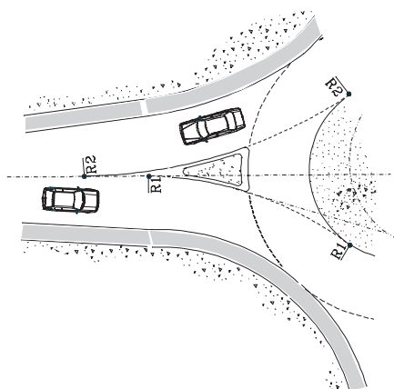
Figura 16 - Traçado do ilhéu separador - zonas com v < 50 \text{ km/h}
