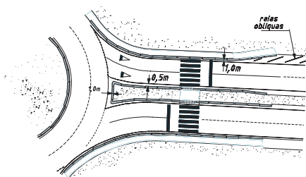
Figura 34 - Definição de passeios em entradas com separador central
