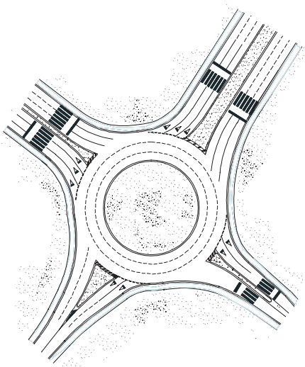
Figura 44 - Marcações rodoviárias - exemplo de aplicação
